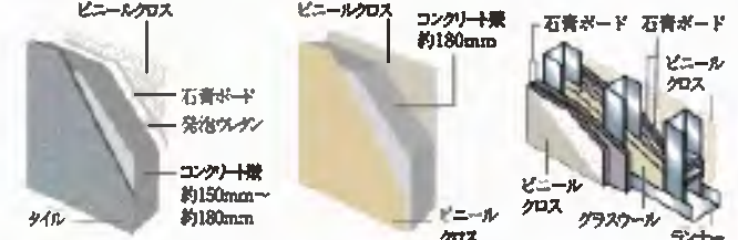
外壁構造図
