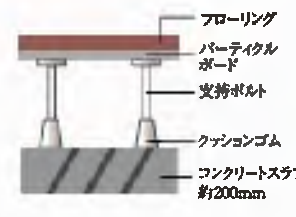
二重床構造図
