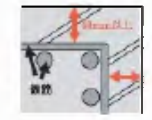
コンクリートかぶり厚断面イメージ図
