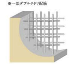
ダブル配筋構造図
