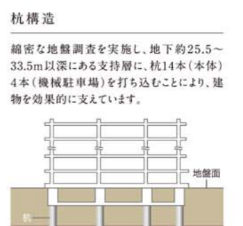
基礎構造概念図
