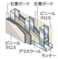
乾式戸境壁構造図
