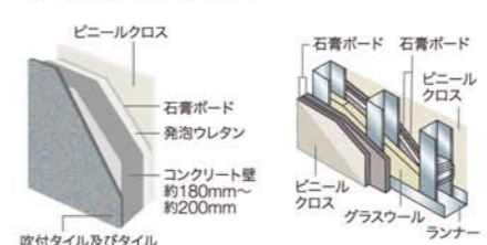
外壁構造図
