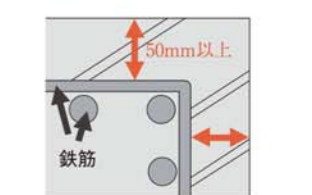
コンクリートかぶり厚断面イメージ図
