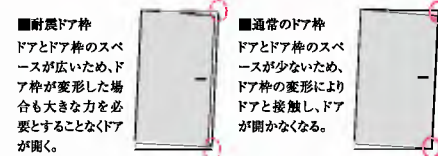
耐震ドア枠
