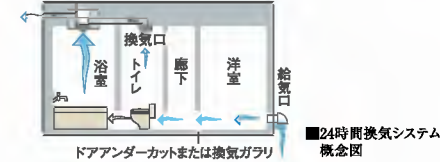
24時間換気システム概念図
