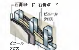
乾式戸境壁構造図
