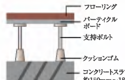
二重床構造図
